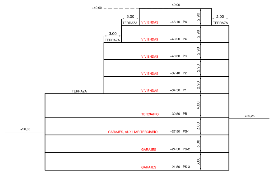
PERFIL NORMATIVO 5.
