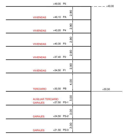
PERFIL NORMATIVO 4.
