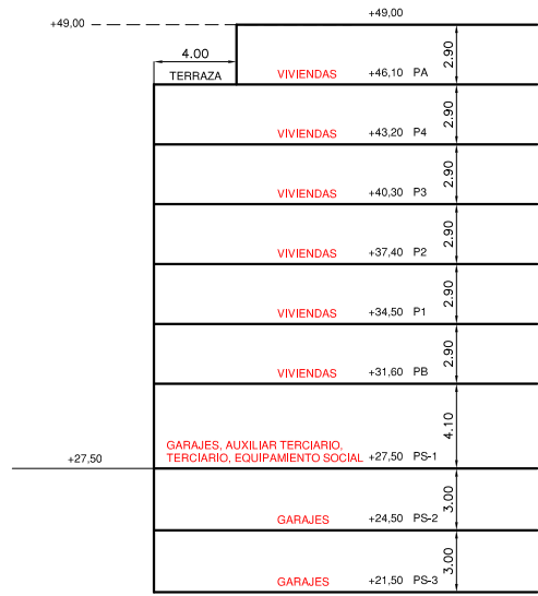
PERFIL NORMATIVO 7.
