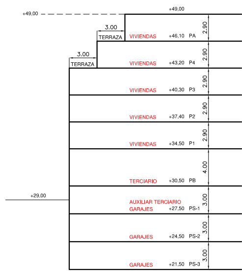
PERFIL NORMATIVO 1.
