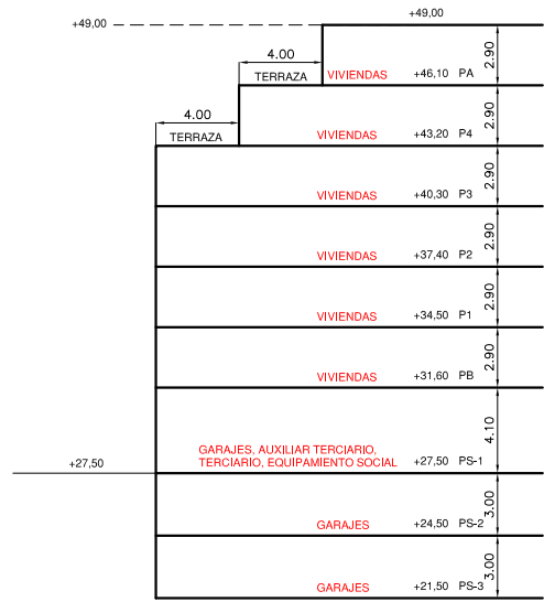
PERFIL NORMATIVO 8.
