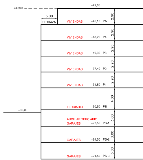
PERFIL NORMATIVO 2.
