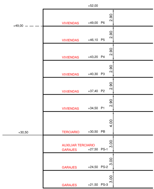
PERFIL NORMATIVO 3.
