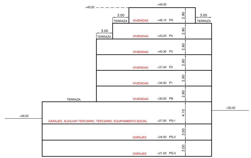
PERFIL NORMATIVO 6.
