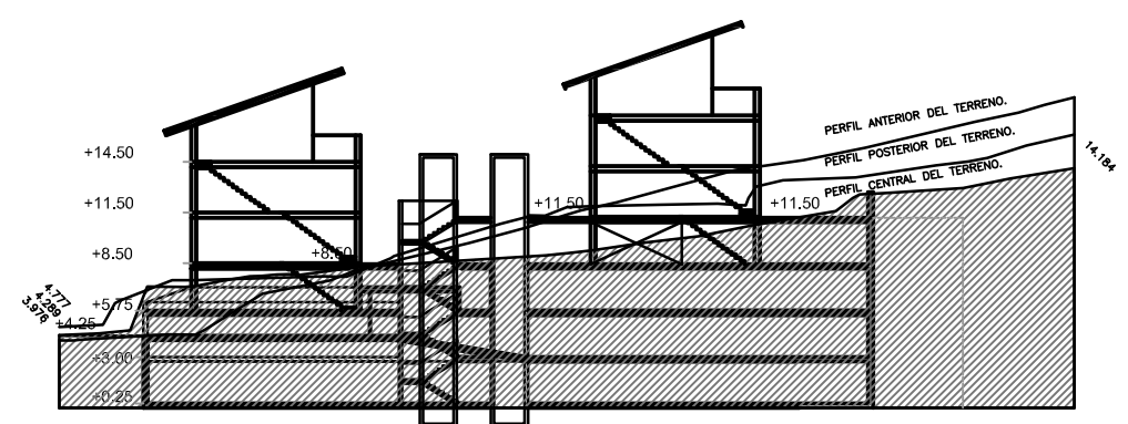
-PROPUESTA ESQUEMATICA DE SECCION TRANSVERSAL-
