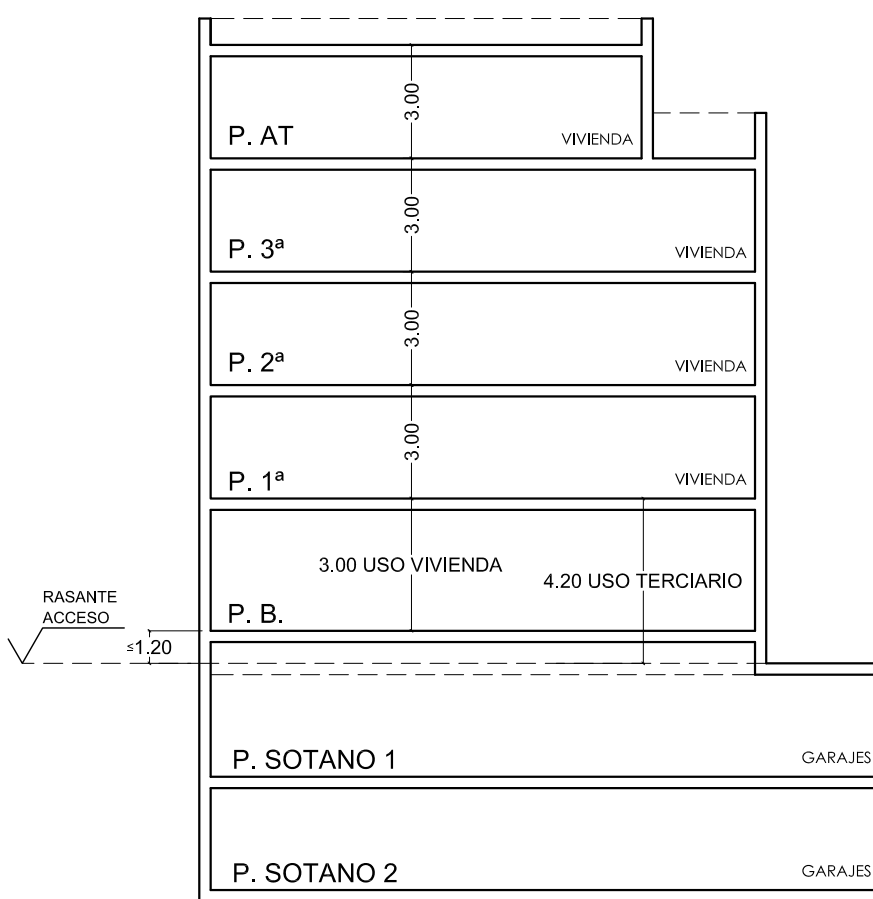
PERFIL NORMATIVO 2 PB+3+AT
