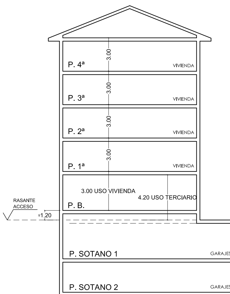
PERFIL NORMATIVO 5 PB+4
