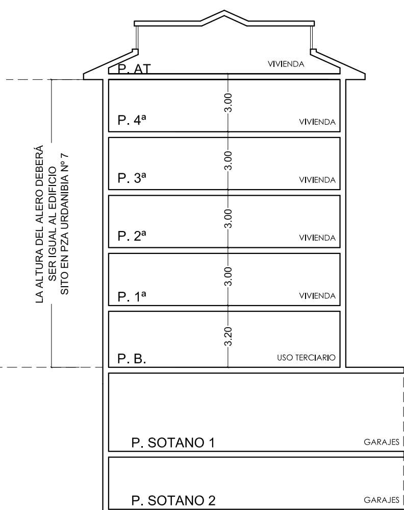
PERFIL NORMATIVO 7 PB+4+AT
