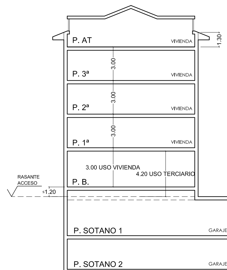
PERFIL NORMATIVO 3 PB+3+AT
