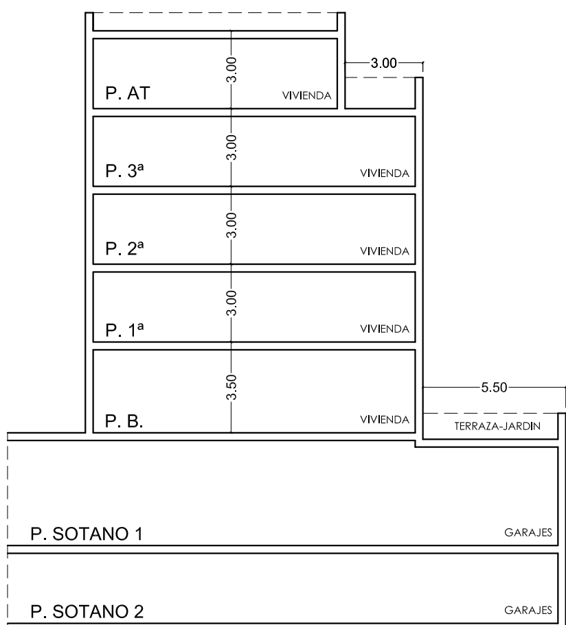
PERFIL NORMATIVO 1 PB+3+AT
