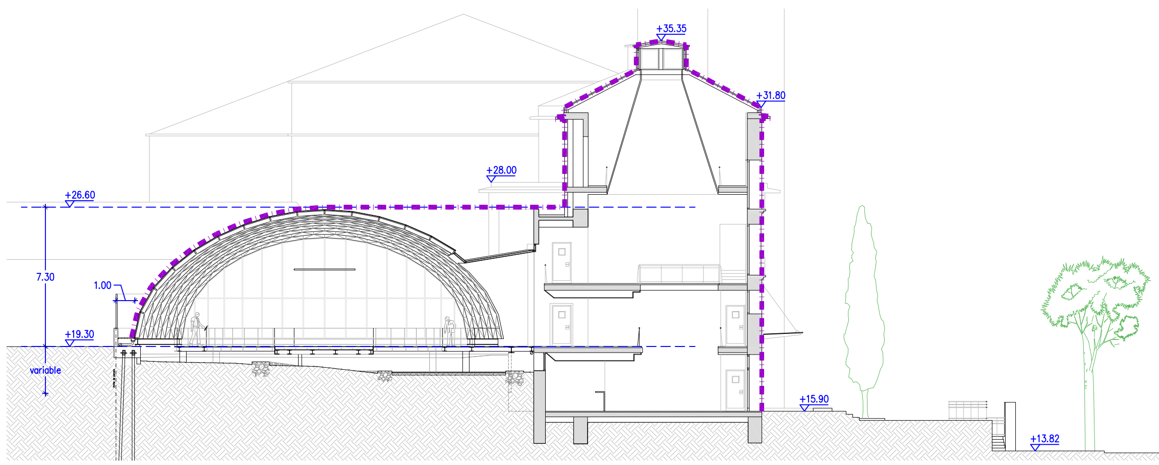
SECCIÓN B
