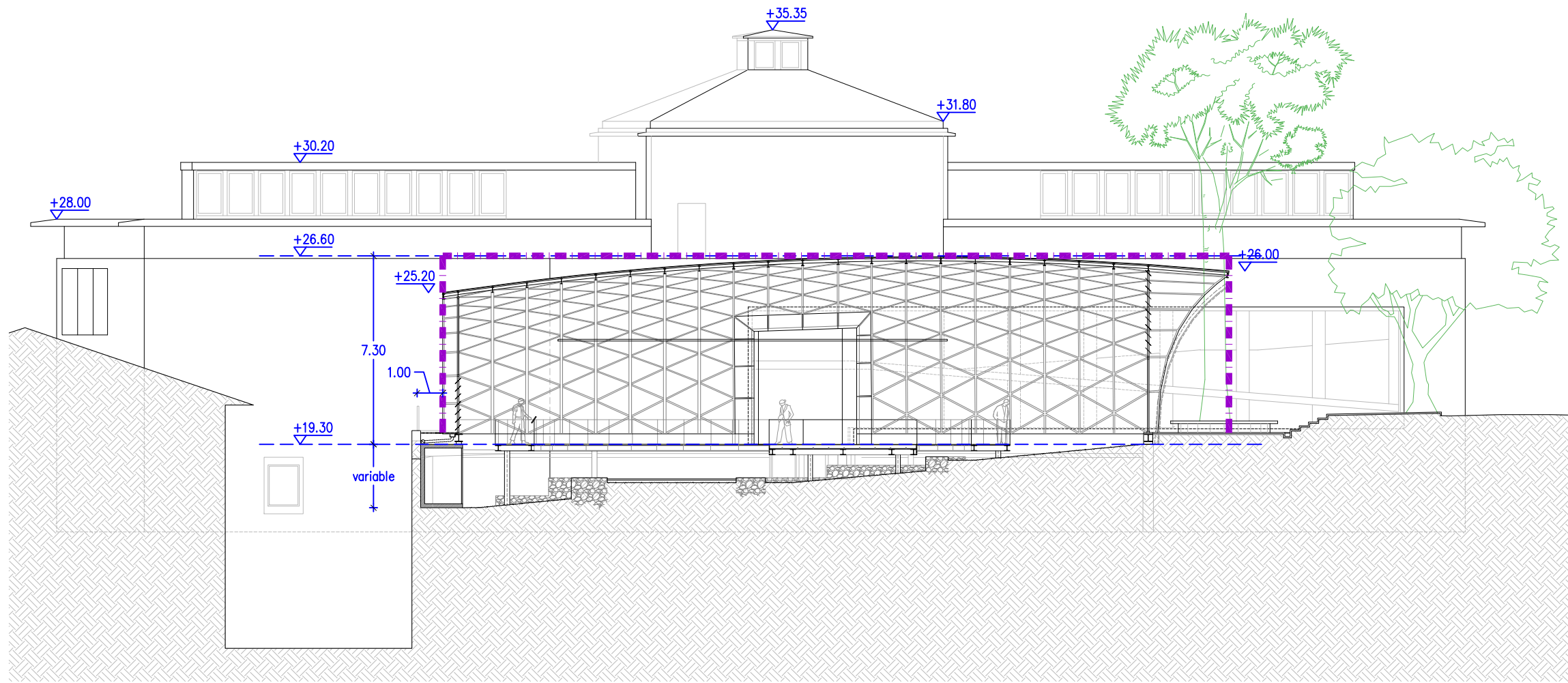
SECCIÓN A
