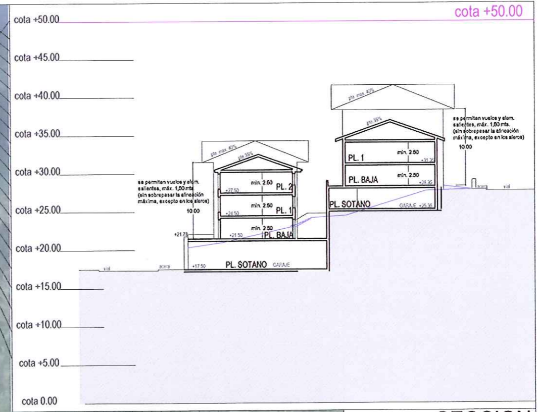
SECCION e: 1/500
